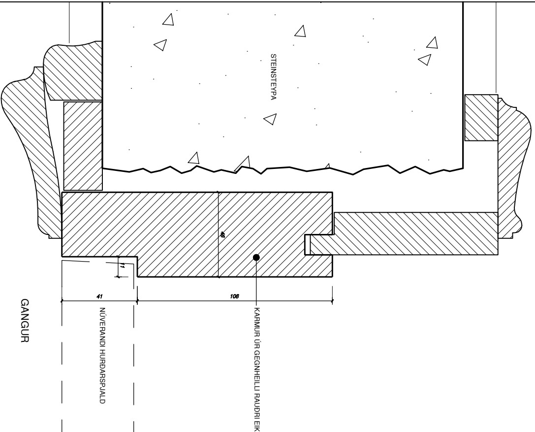
A 32/02 NÚVERANDI FYRIRKOMULLAG LARÉTTI SNID MÁL 1:1
